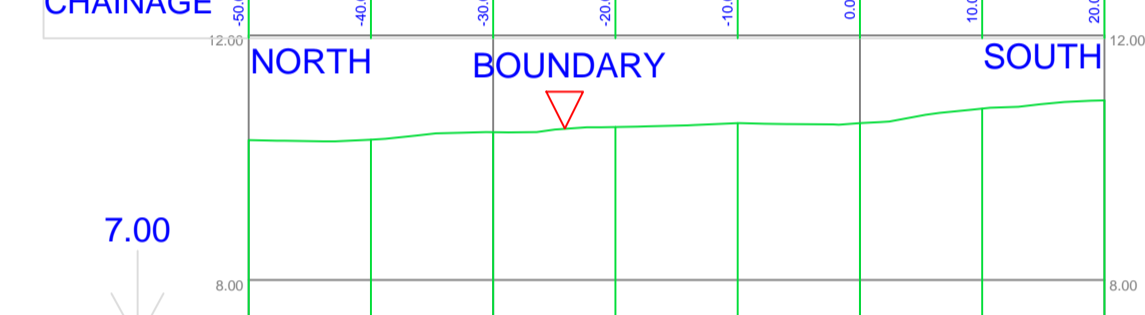
SECTION D 90.000 Horiz. 1:500 Vert. 1:100
