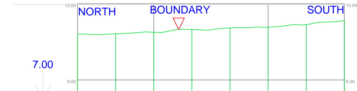
SECTION E 120.000 Horiz. 1:500 Vert. 1:100
